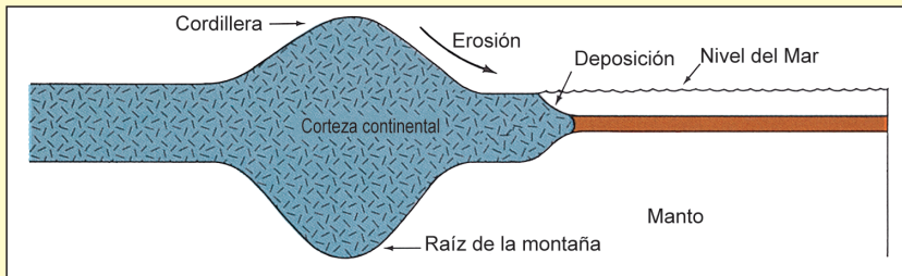
Figura 9: Otra ilustración muestra cómo las montañas tienen forma de "estaca", debido a sus profundas raíces. ( Earth Science [Ciencia de la Tierra] , Tarbuck y Lutgens, p. 157.)
