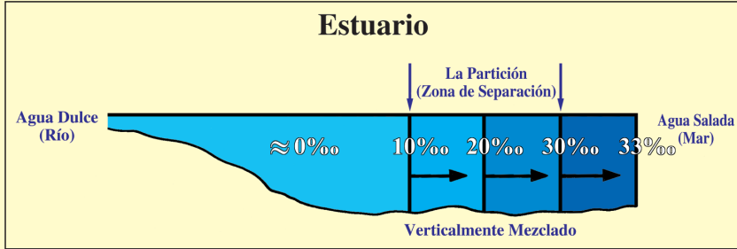
Figura 14: Corte longitudinal que muestra la salinidad (partes por mil ‰), en un estuario. Aquí podemos observar la partición (Zona de separación), entre el agua dulce y la salada. (Levemente modificado de Introductory Oceanography [Oceanografía Introductoria], Thurman, p. 301.)
