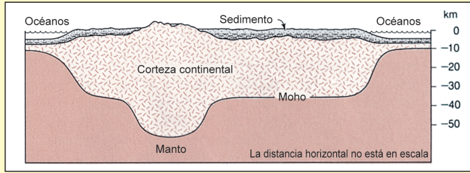
Figura 7: Las montañas tienen profundas raíces bajo la superficie terrestre. ( Earth [La Tierra] , Press y Siever, p. 413.)
